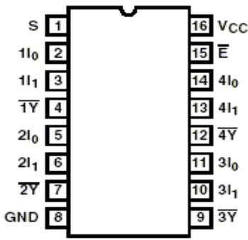
外引线排列
