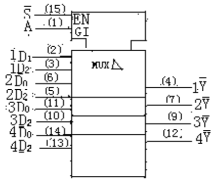
逻辑符号
