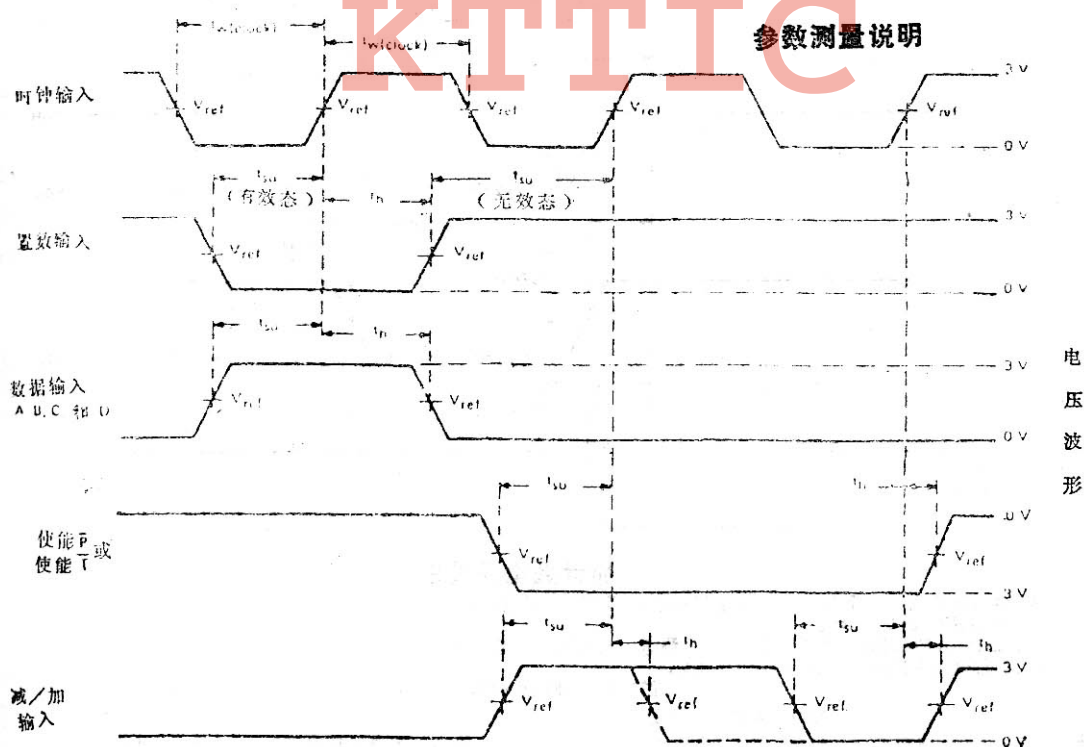
图1 时钟输入、置数输入和使能输入
