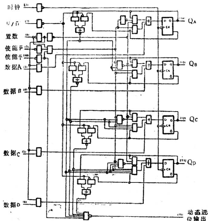
逻辑图
