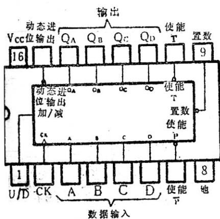
外引线排列图
