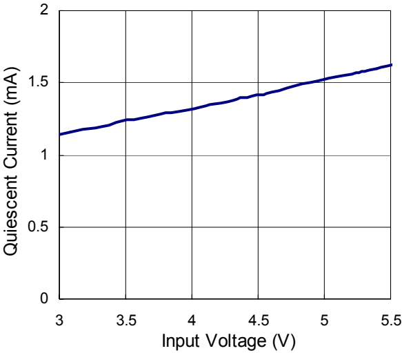
Quiescent Current vs. VIN (Switching)
