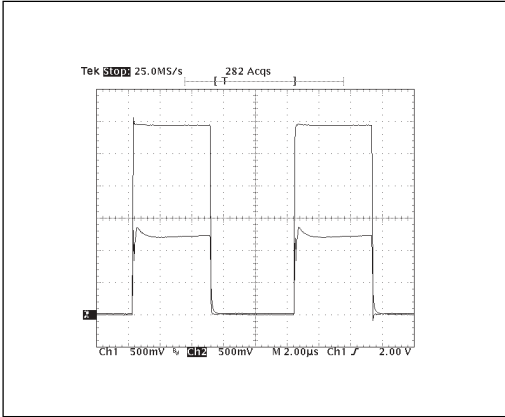
I KA = 0 to 1mA.
