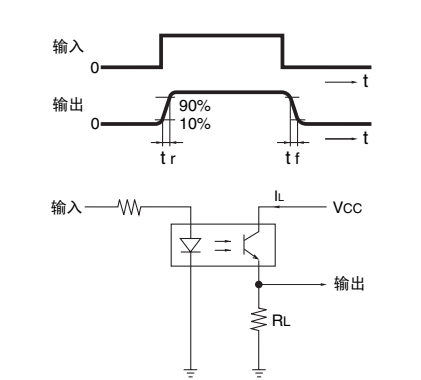
图 10. 应答时间测定回路
