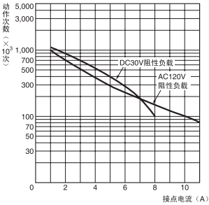
●寿命曲线
