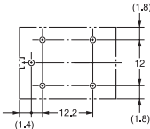
底视端子安装图
