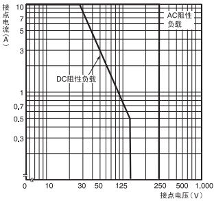
●开关容量的最大值
