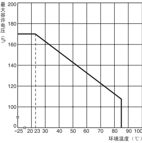
●环境温度与最大容许电压
