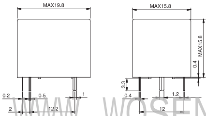
单刀单掷一常开
