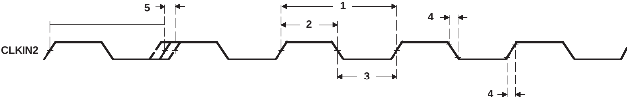
Figure 7-30. CLKIN2 Timing
